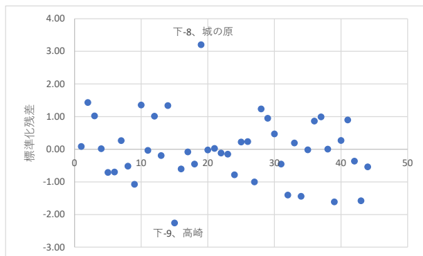
図4 標準化残差
